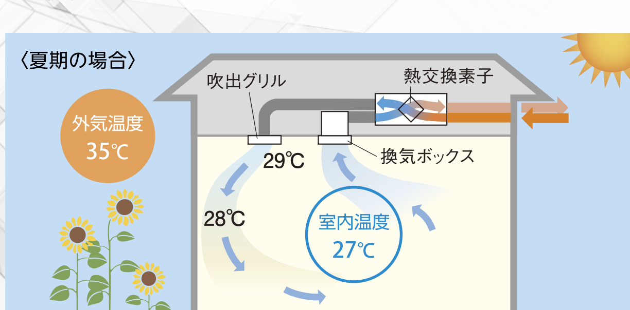
温度交換効率75%の場合のイメージ図
